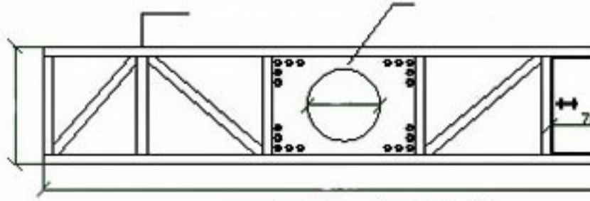
KASET İÇİ ÜST GÖRÜNÜŞÜ
